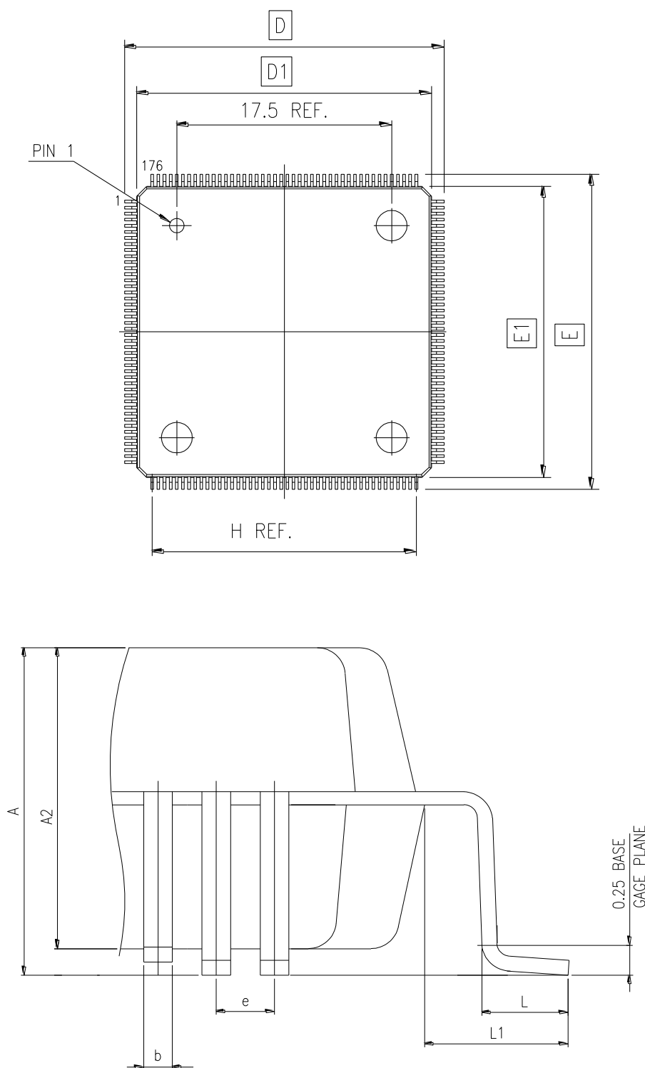
图 16 LQFP176 封装图
